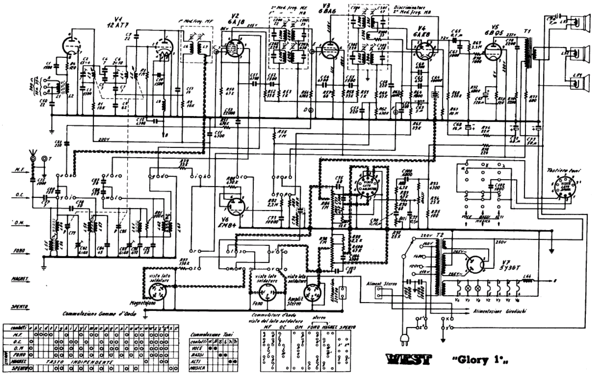
WEST RADIO-TV - Mod. GLORY 1°. Radiofonografo AM/FM a sei valvole più occhio magico. Antenne per AM e FM incorporate. Media frequenza AM a 455 kc/s, media frequenza FM a 10,7 Mc/s. Potenza d'uscita 5 watt. Consumo 80 watt.
